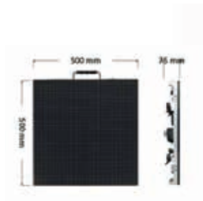
DALLE P3,9 DE 0,5M
