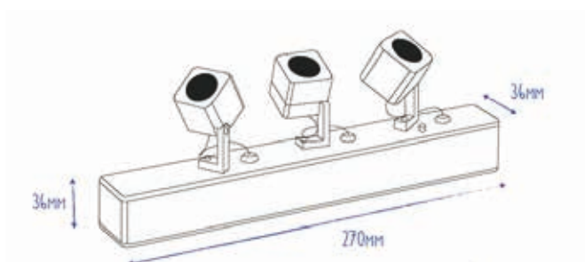
ÉCLAIRAGE MOBILE PAK
